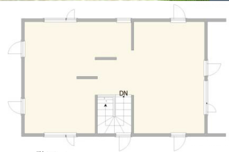
2階平面図
